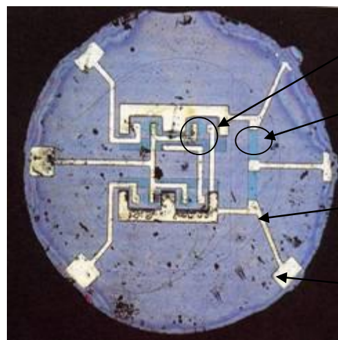
Увеличенная фотография первой планарной микросхемы
